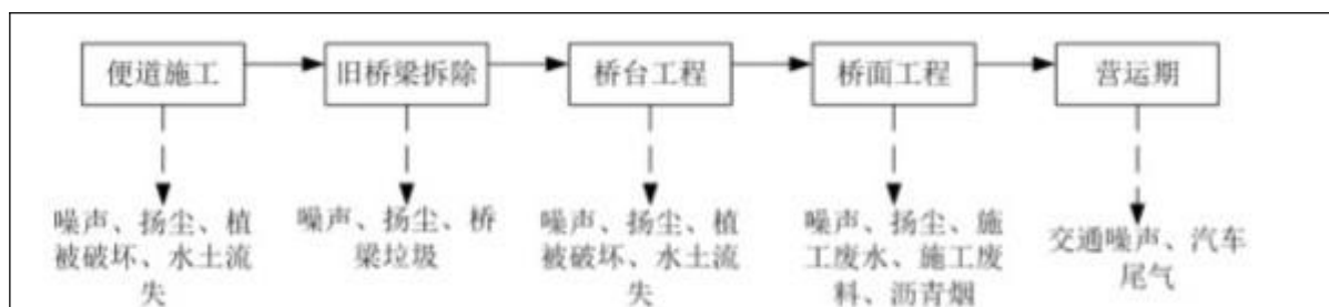
图 5-1 施工期、营运期工程工艺流程及产污流程图
