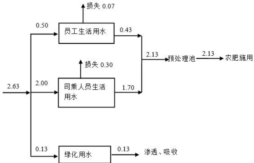
图 3-1 本项目水平衡 (t/d)
