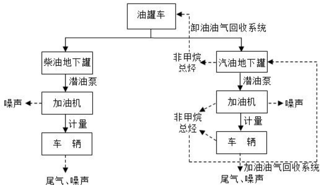
图 2-1 加油生产工艺及产污位置示意图
