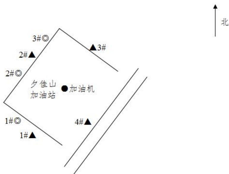
图例：◎无组织废气采样点 ▲噪声检测点 ●噪声源
